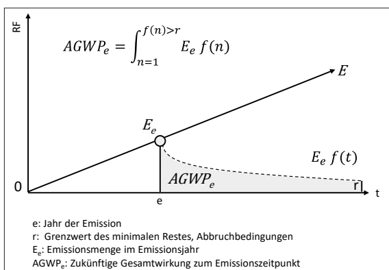
Abbildung 4: Berechnung von AGWP e nach Myhre et al. 2013
