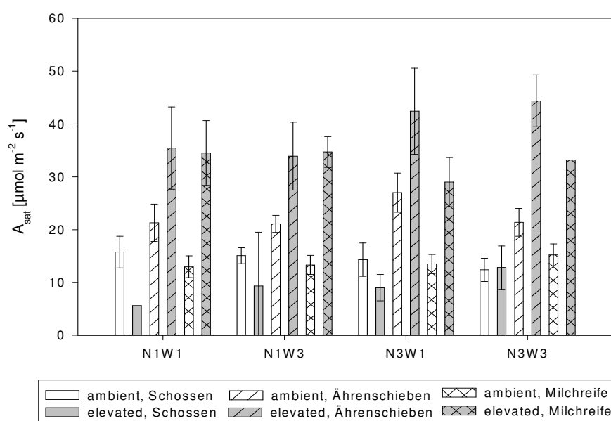
Abb. 2.: Lichtgesättigte Photosyntheserate ( A_{\text{sat}} ) im Verlauf der Entwicklung (Konfidenzintervall: 90%).
