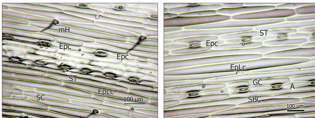
Abb. 5 Abdrücke der Blattoberseite (links) und Blattunterseite (rechts) der optimal wasserversorgten (W3) und gut stickstoffversorgten (N3) Pflanzen im Stadium des Schossens, (Vergrößerung: 100x);
