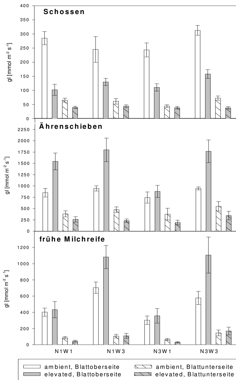
Abb. 6.: Darstellung der Blattleitfähigkeit (Wochenmittelwerte) der verschiedenen Versuchsansätze unter derzeitigen klimatischen Verhältnissen und erhöhter atmosphärischer CO 2 -Konzentration und Temperatur im Verlauf der Entwicklung, (Konfidenzintervall: 90%).
