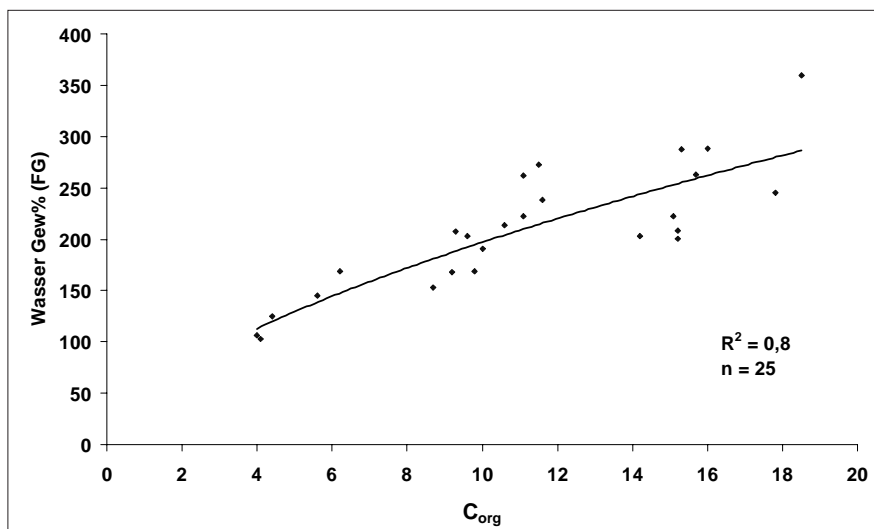
Abbildung 9: Beziehung zwischen C_{org} und Wasserspeicherkapazität von Gebirgsböden; FG = Fließgrenze
