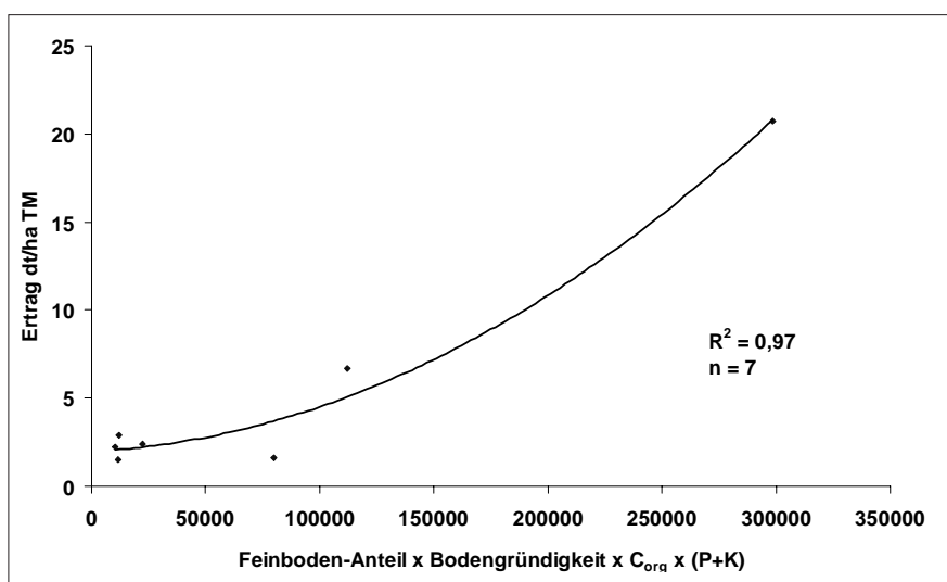
Abbildung 12: Beziehung zwischen (Feinboden-Anteil x Bodengründigkeit x C_{org} x (P+K)) und Ertrag
