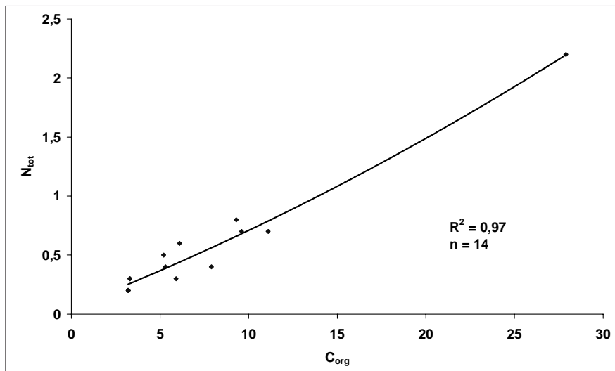
Abbildung 8: Beziehung zwischen C_{org} und N_{tot}
