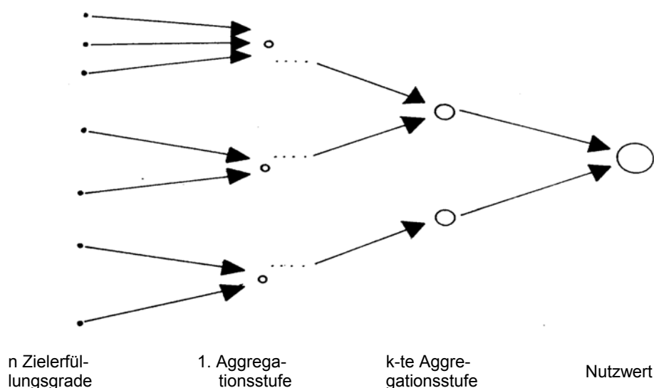
Abbildung 2.2: Schrittweise Wertsynthese
