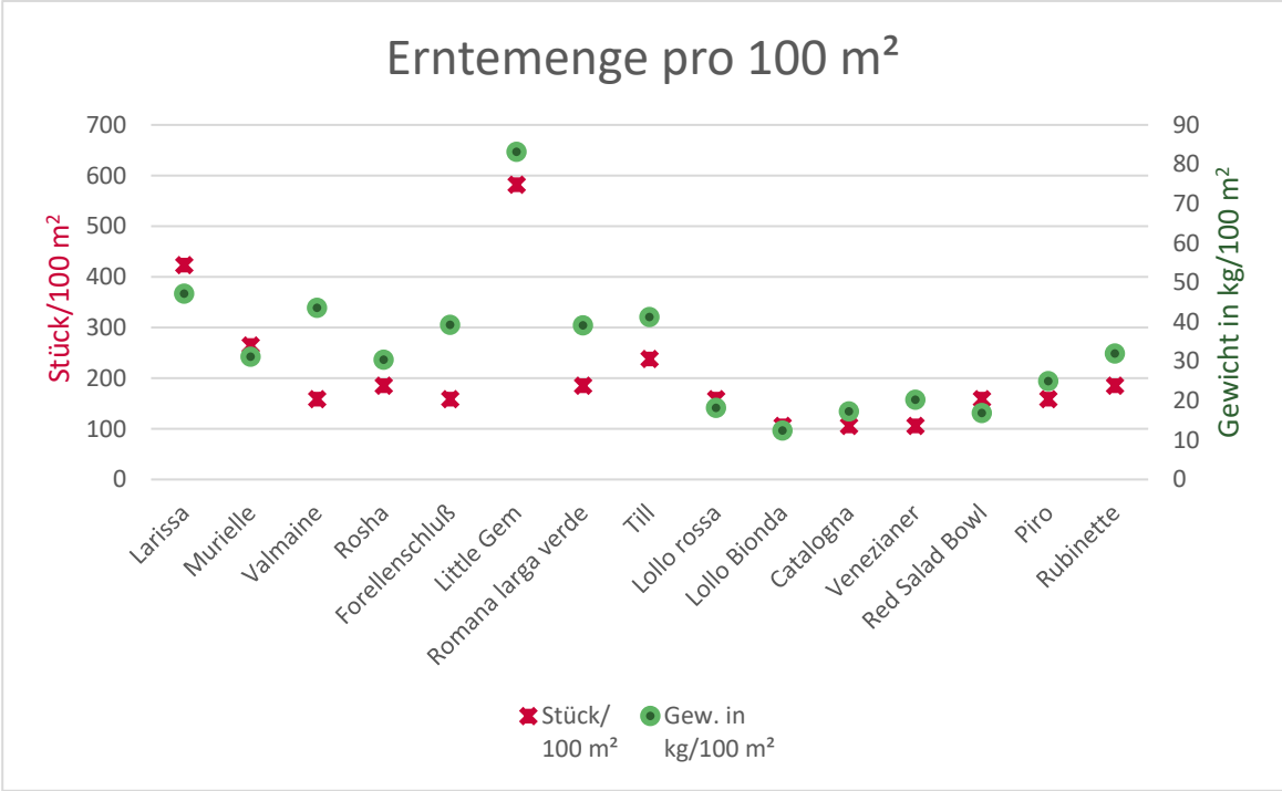
Abb. 2: Ertragsergebnisse des kalten Salat-Sortenversuchs im Glashaus, marktfähige Ware (Außenstelle Zinsenhof), Stückertrag pro 100 m 2 , Gewichtsertrag in kg pro 100 m 2
