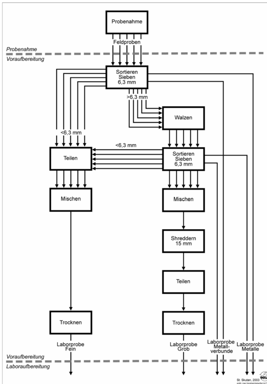
Abbildung 4-31: Schema der Voraufbereitung für die Proben der Feinfraktion <50 mm. Die jeweils fünf parallelen Pfeile geben nicht eine Probenanzahl wieder, sondern symbolisieren, dass die Schritte bis zum Mischen mit vielen Einzelproben (in zeitlichem Abstand) separat durchlaufen werden. In diesem System wird physisch keine Mischprobe als Summe aller gezogenen Einzel-Feldproben erzeugt, sondern die Mischprobenbildung erfolgt erst mit den voraufbereiteten und geteilten Einzelproben.
