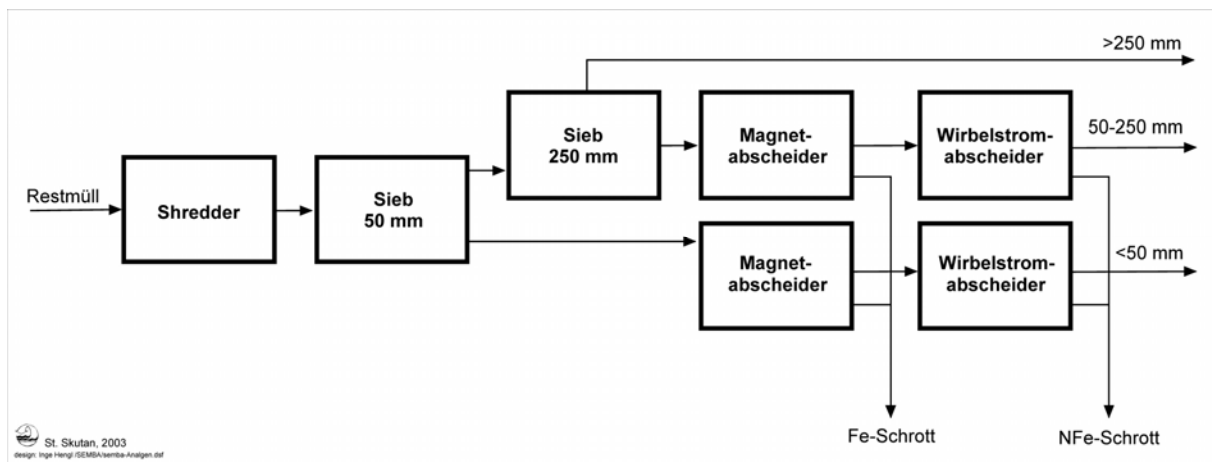
Abbildung 4-35: Schema der Splittinganlage Wien (Anmerkung: Der Übersichtlichkeit wegen ist die doppelte Magnetscheidung mit Kopftrommel- und Überbandmagnet bei der Fraktion <50 mm nicht eingezeichnet.)
