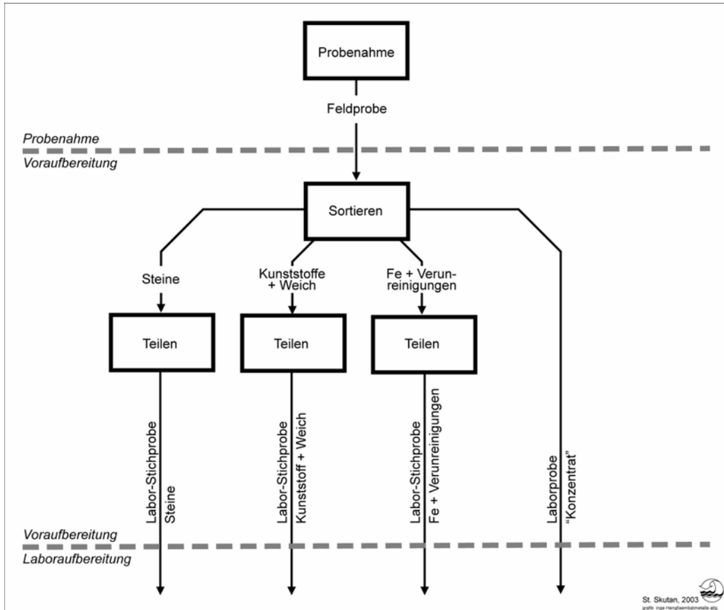
Abbildung 3-31: Allgemeines Schema für die Voraufbereitung von Metallschrottpollen am Ort der Probenahme
