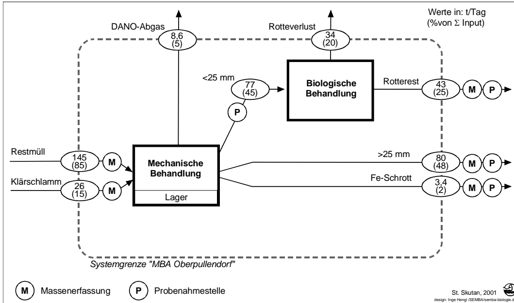
Abbildung 4-3: Systembild für die Stoffflussanalyse an der MBA Oberpullendorf Hauptversuch (Versuch „Oberpullendorf I“): Vorabschätzung der Güterflüsse für die Versuchsplanung in t/Tag bzw. % von der Summe Input (Restmüll + Klärschlamm); ebenfalls eingezeichnet sind die Stellen für Massenerfassung und Probenahme
