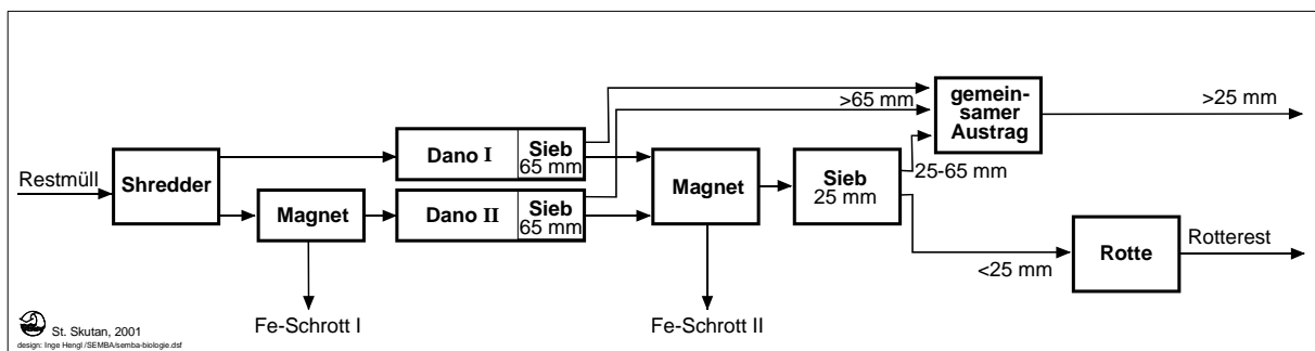
Abbildung 4-1: Anlagenschema der MBA Oberpullendorf (Stand 2001) bei stillgelegter Aufbereitung der Mittelfraktion 25-65 mm (Versuch „Oberpullendorf I“)
