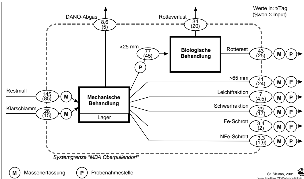
Abbildung 4-4: Systembild für die Stoffflussanalyse an der MBA Oberpullendorf unter geänderten Bedingungen (Versuch „Oberpullendorf II“): Vorabschätzung der Güterflüsse für die Versuchsplanung in t/Tag bzw. % von der Summe Input (Restmüll + Klärschlamm); ebenfalls eingezeichnet sind die Stellen für Massenerfassung und Probenahme
