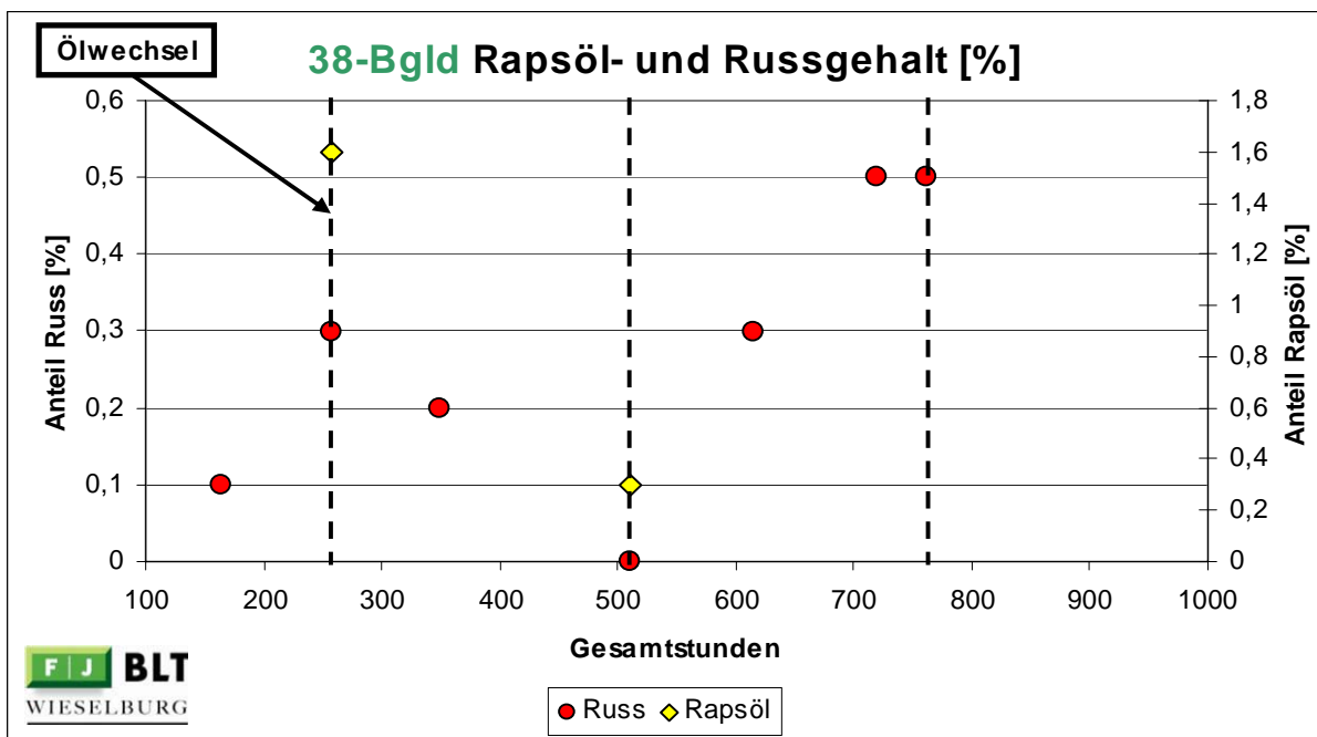
Abbildung 174: 38-Bgld Rapsöl- und Russgehalt in den Motorölproben
