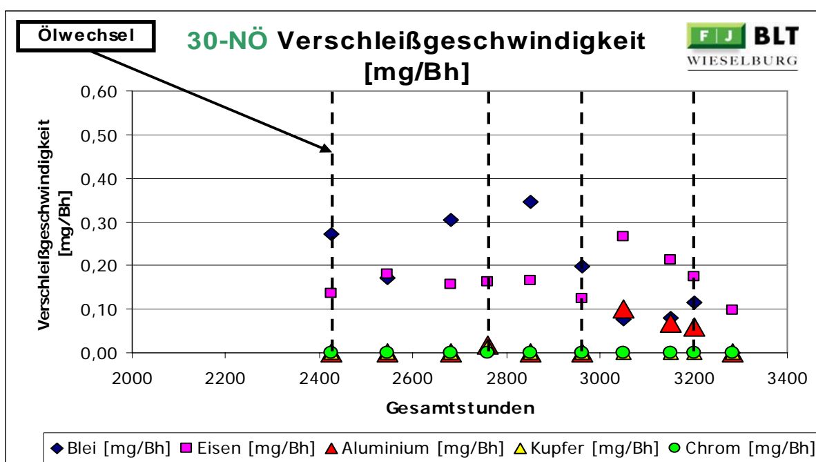
Abbildung 45: 30-NÖ Verschleißgeschwindigkeit
