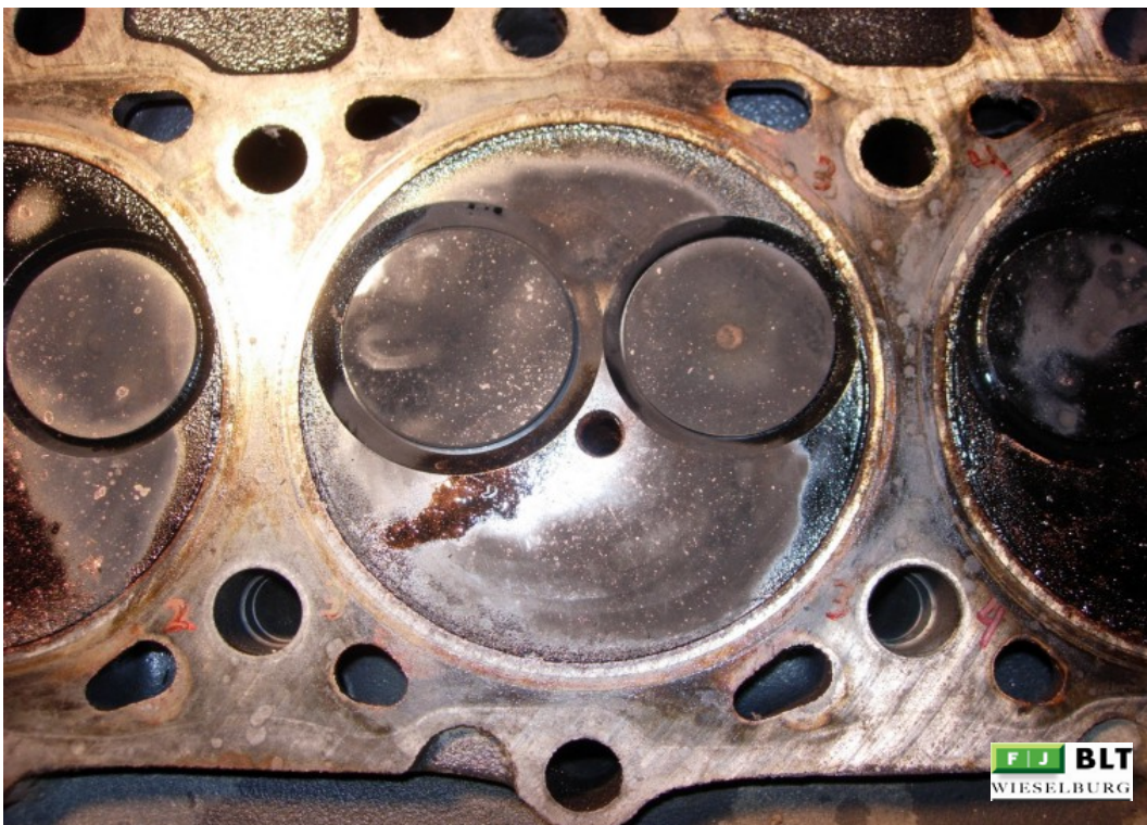
Abbildung 176: 38-Bgld Zylinderkopf
