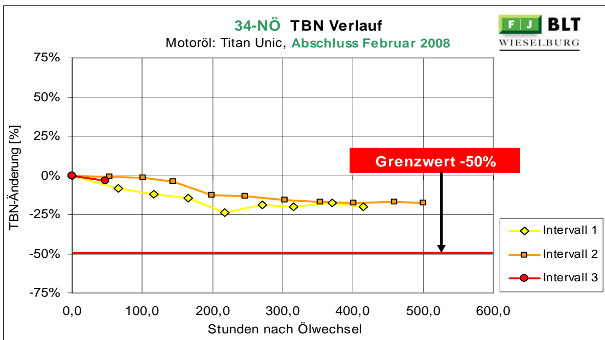
Abbildung 112: 34-NÖ Änderung der Total Base Number
