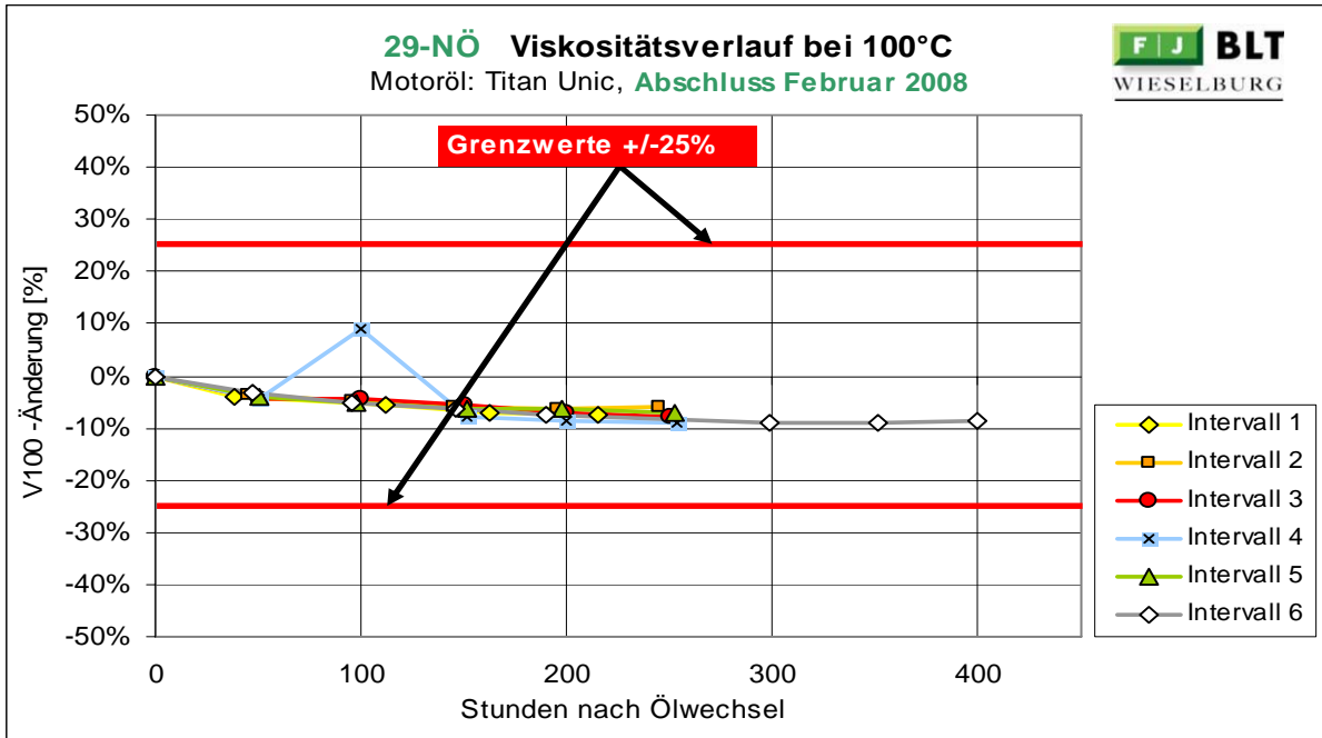
Abbildung 28: 29-NÖ Änderung der Viskosität bei 100°C
