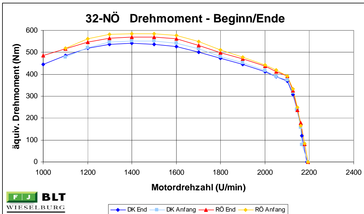
Abbildung 74: 32-NÖ Äquiv. Drehmoment Dieselkraftstoff und Rapsöl Beginn/Ende
