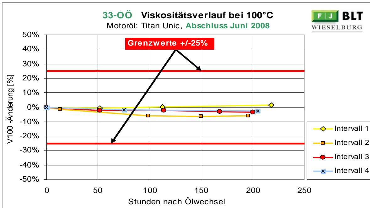
Abbildung 95: 33-OÖ Änderung der Viskosität bei 100°C
