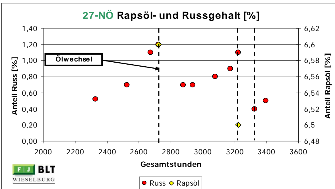
Abbildung 10: 27-NÖ Rapsöl- und Russgehalt in den Motorölproben
