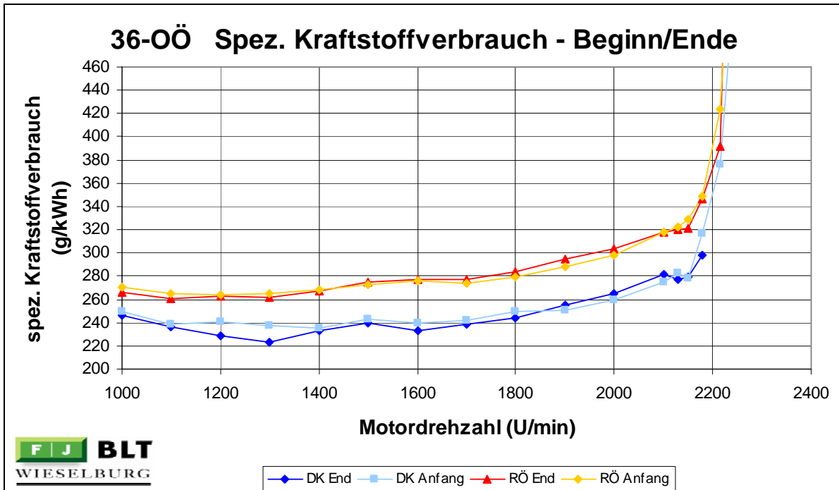
Abbildung 134: 36-OÖ Spezifischer Kraftstoffverbrauch Dieselkraftstoff und Rapsöl Beginn/Ende
