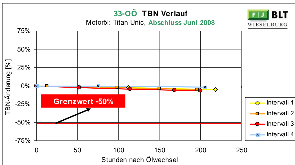
Abbildung 96: 33-OÖ Änderung der Total Base Number
