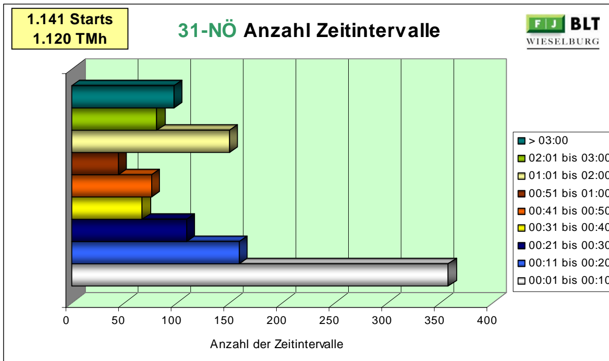
Abbildung 63: 31-NÖ Zeitintervalle aufgetragen auf die Anzahl der Starts
