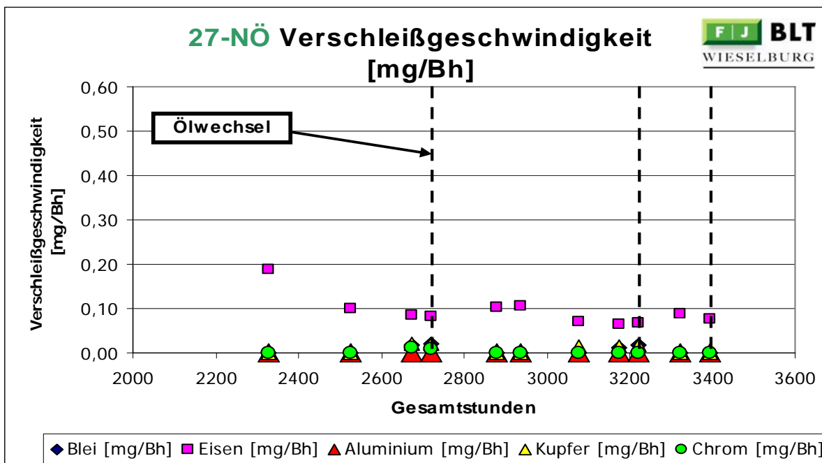
Abbildung 9: 27-NÖ Verschleißgeschwindigkeit [mg/Bh]
