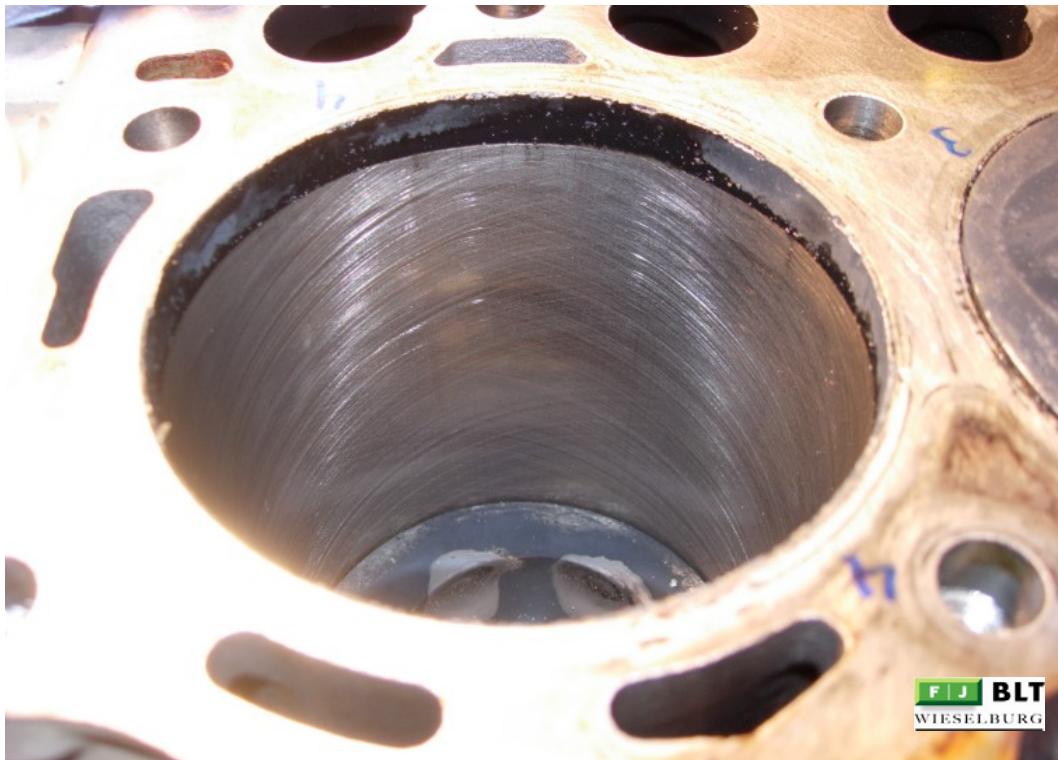
Abbildung 35: 29-NÖ Zylinderlaufbüchse
