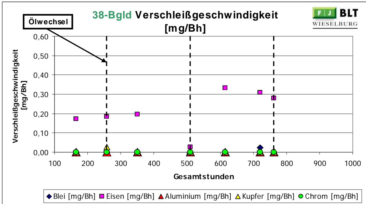
Abbildung 173: 38-Bgld Verschleißgeschwindigkeit
