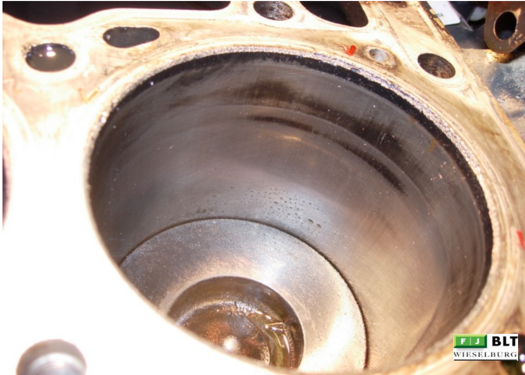
Abbildung 178: 38-Bgld Zylinderlaufbüchse
