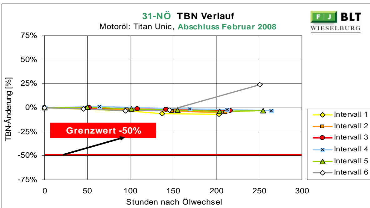
Abbildung 59: 31-NÖ Änderung der Total Base Number
