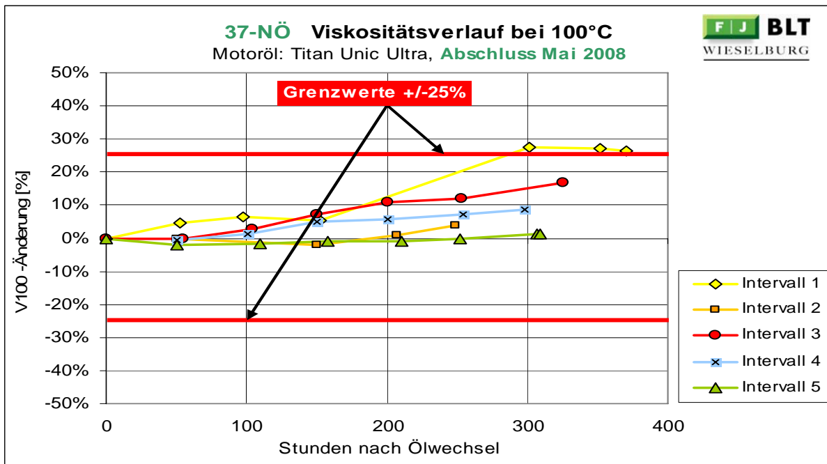
Abbildung 154: 37-NÖ Änderung der Viskosität bei 100°C
