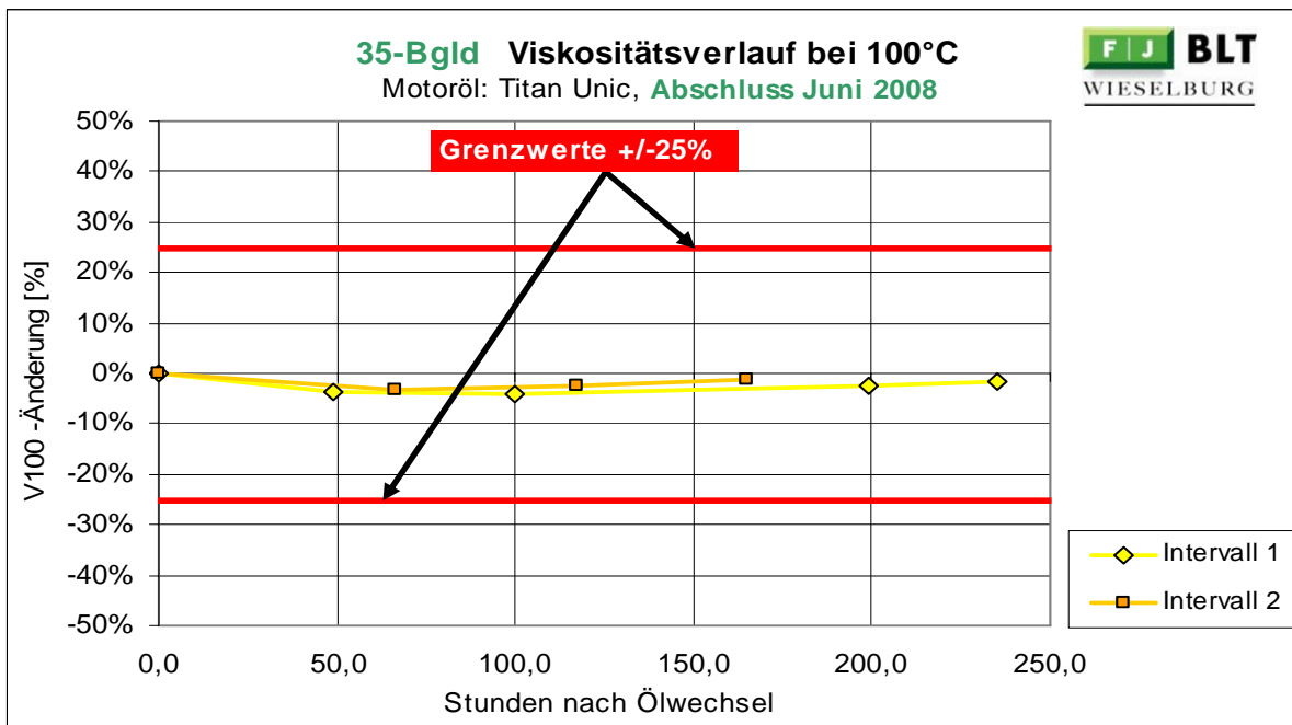
Abbildung 127: 35-Bgld Änderung der Viskosität bei 100°C
