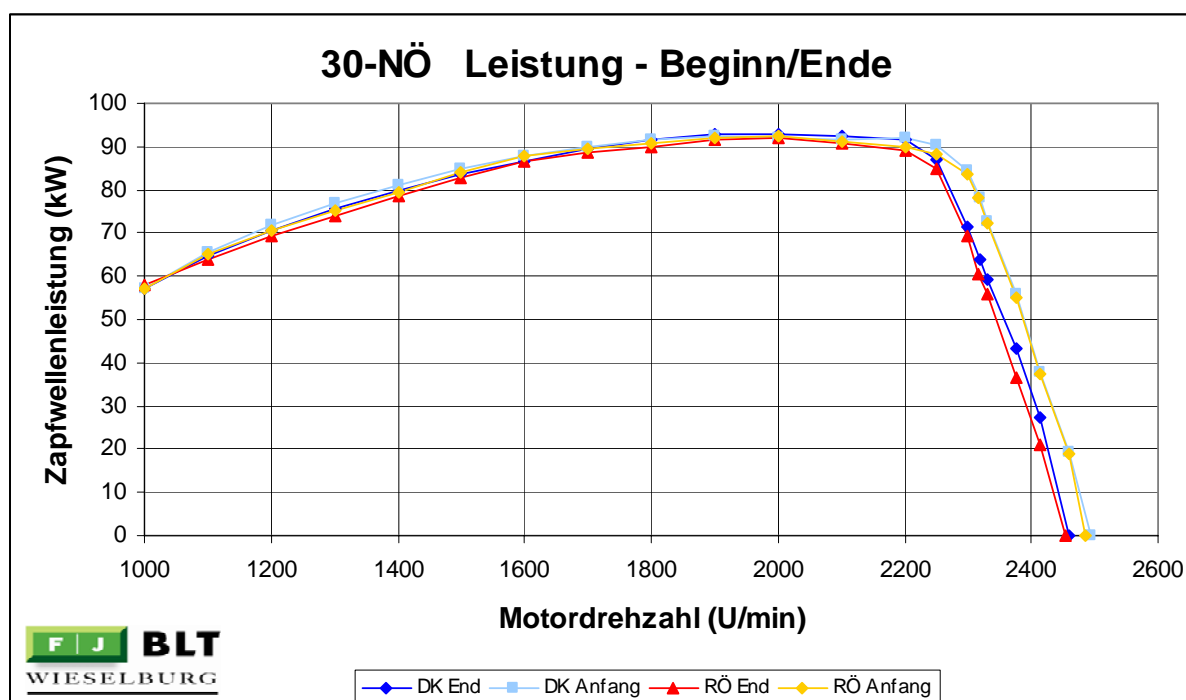
Abbildung 37: 30-NÖ Zapfwellenleistung Dieselkraftstoff und Rapsöl Beginn/Ende
