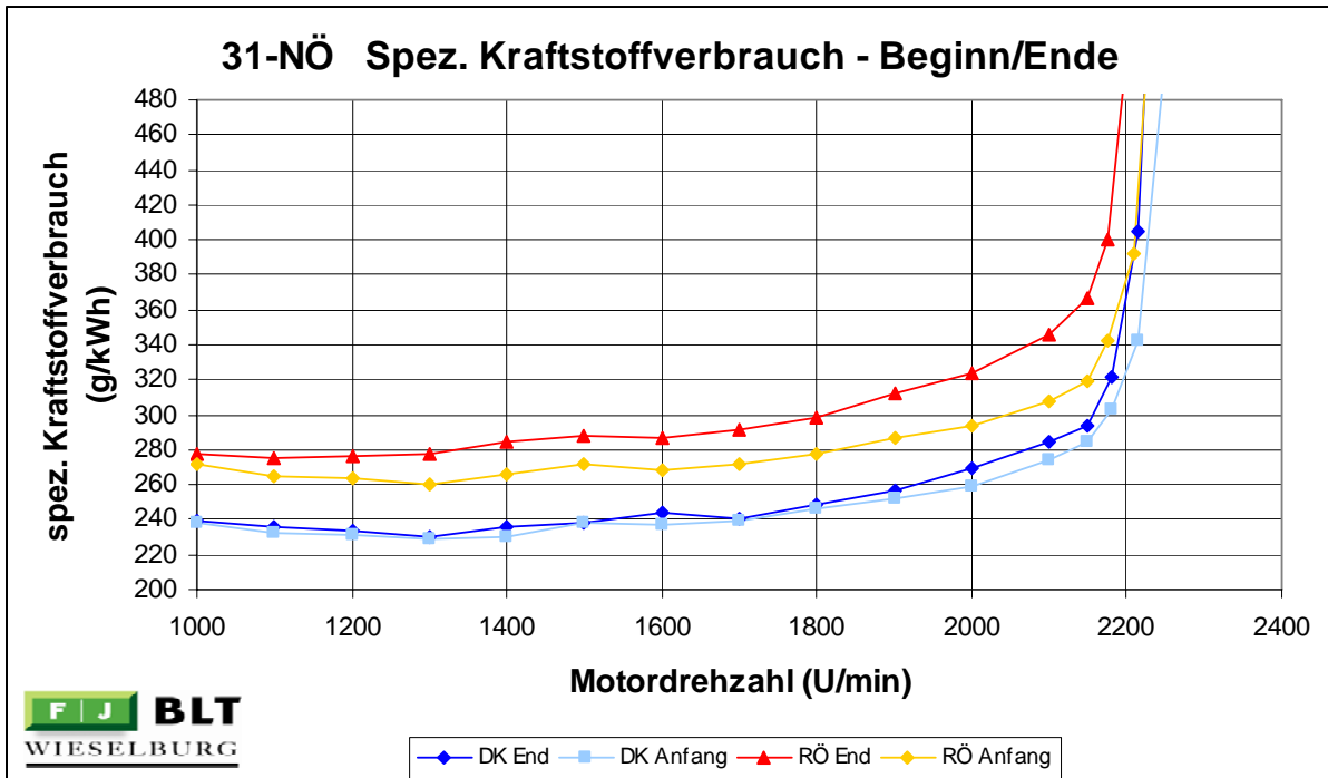
Abbildung 55: 31-NÖ Spezifischer Kraftstoffverbrauch Dieselkraftstoff und Rapsöl Beginn/Ende
