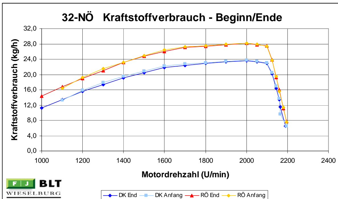
Abbildung 75: 32-NÖ Kraftstoffverbrauch Dieselkraftstoff und Rapsöl Beginn/Ende
