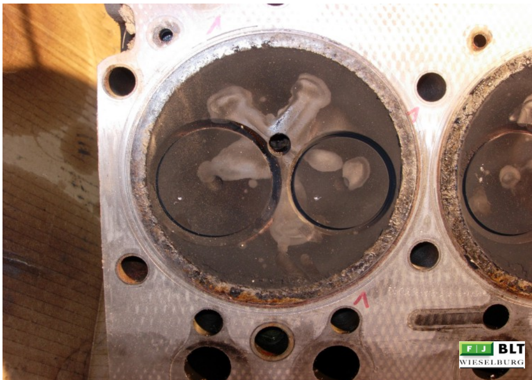
Abbildung 69: 31-NÖ Zylinderkopf
