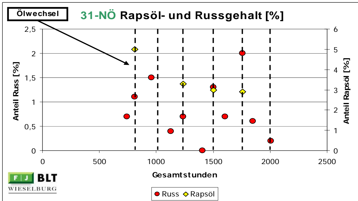
Abbildung 61: 31-NÖ Rapsöl- und Russgehalt in den Motorölproben
