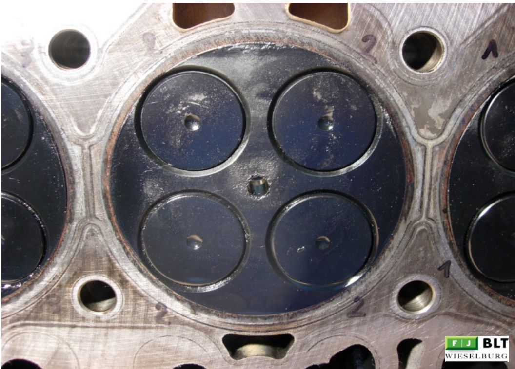
Abbildung 84: 32-NÖ Zylinderkopf
