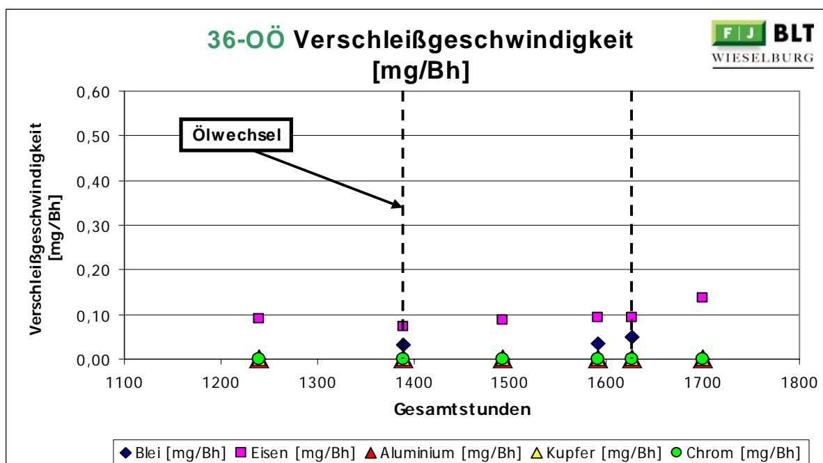
Abbildung 139: 36-OÖ Verschleißgeschwindigkeit
