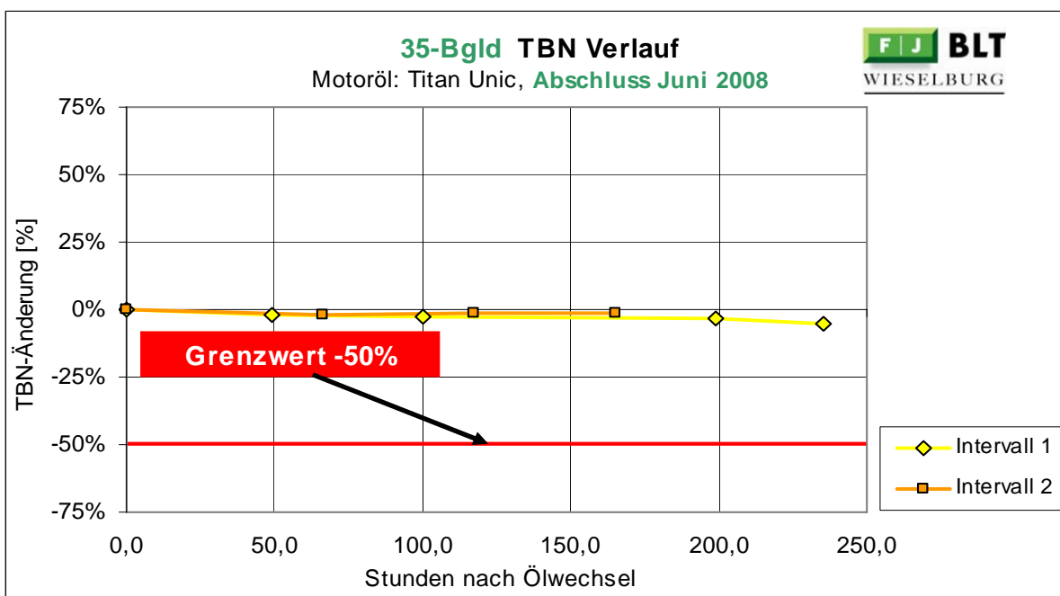
Abbildung 128: 35-Bgld Änderung der Total Base Number
