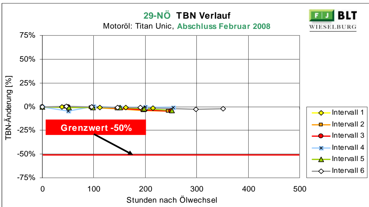
Abbildung 29: 29-NÖ Änderung der Total Base Number
