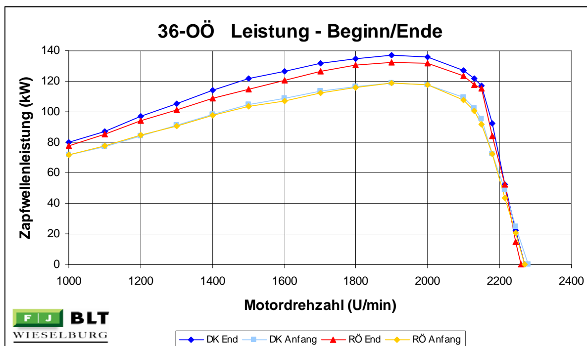
Abbildung 131: 36-OÖ Zapfwellenleistung Dieselkraftstoff und Rapsöl Beginn/Ende
