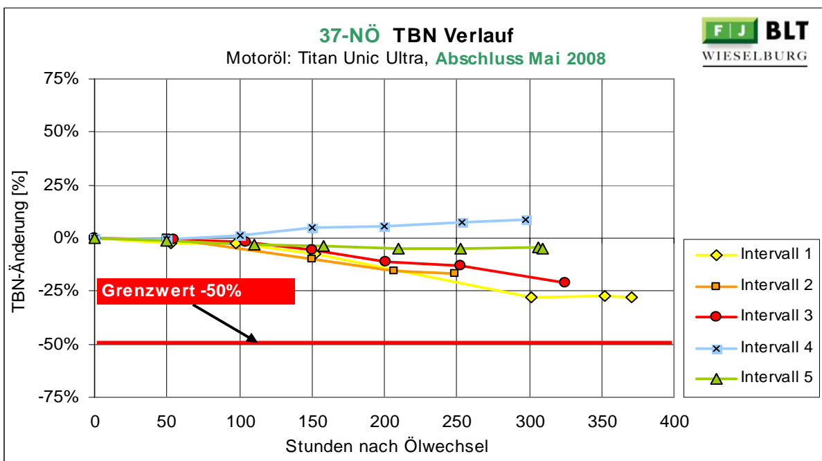
Abbildung 155: 37-NÖ Änderung der Total Base Number
