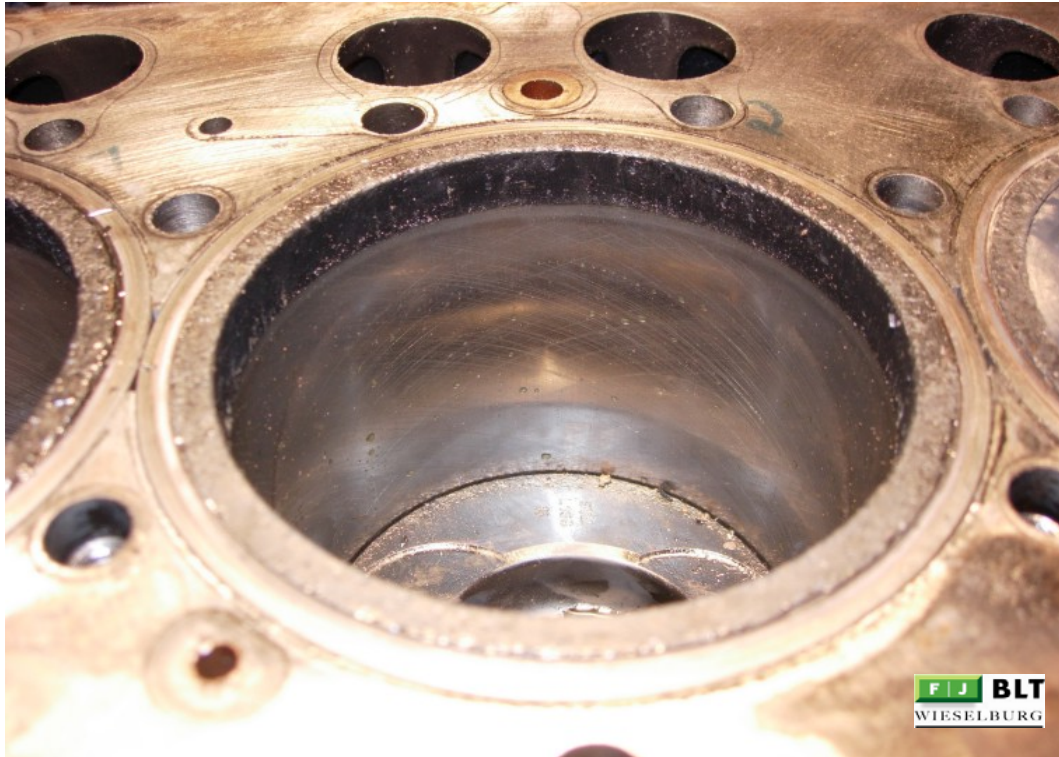
Abbildung 50: 30-NÖ Zylinderlaufbüchse
