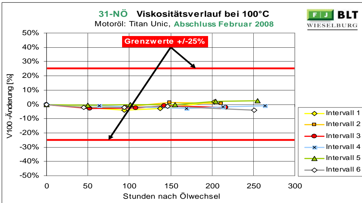
Abbildung 58: 31-NÖ Änderung der Viskosität bei 100°C
