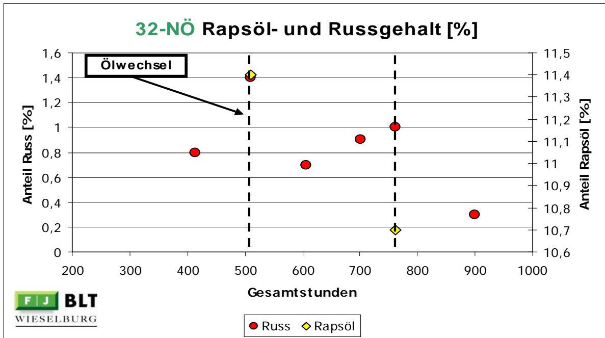
Abbildung 82: 32-NÖ Rapsöl- und Russgehalt in den Motorölproben
