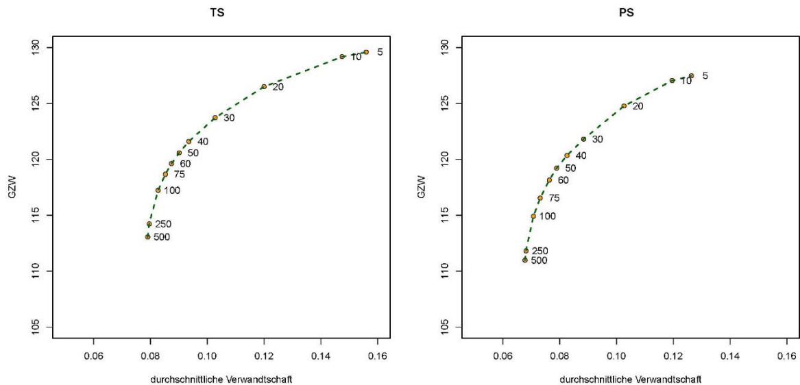
Abbildung 7: Verhältnis von durchschnittlicher Verwandtschaft der angepaarten Tiere zu deren Gesamtzuchtwert bei unterschiedlichem Gewichtungsfaktor im Teststiermodell (TS, links) und Altstiermodell (PS, rechts)
