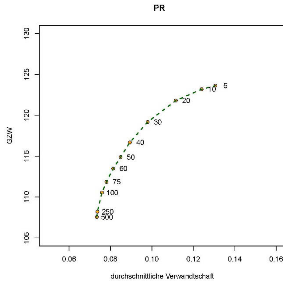
Abbildung 4: Verhältnis von durchschnittlicher Verwandtschaft der angepaarten Tiere zu deren Gesamtzuchtwert bei unterschiedlichem Gewichtungsfaktor in der Altstiervariante (PR)
