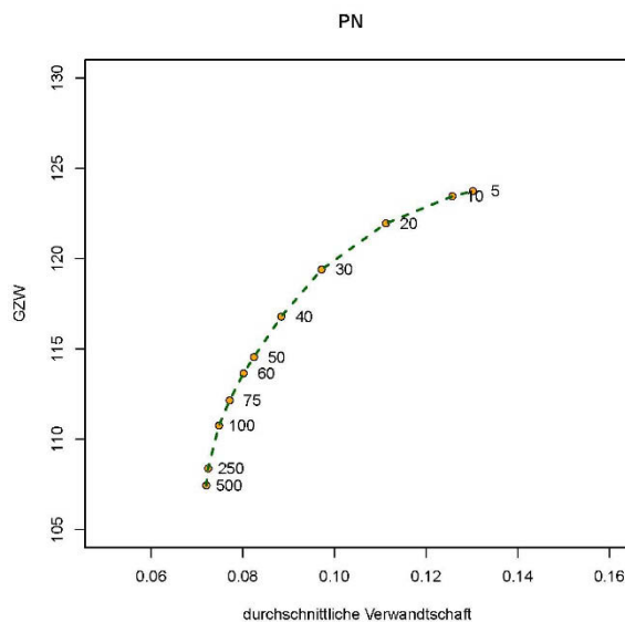
Abbildung 6: Verhältnis von durchschnittlicher Verwandtschaft der angepaarten Tiere zu deren Gesamtzuchtwert bei unterschiedlichem Gewichtungsfaktor im Altstiermodell (PN)
