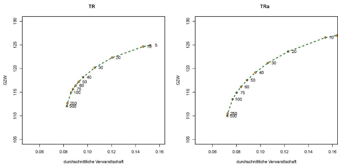
Abbildung 3: Verhältnis von durchschnittlicher Verwandtschaft der angepaarten Tiere zu deren Gesamtzuchtwert bei unterschiedlichem Gewichtungsfaktor in der Teststiervariante (TR, links) und der erweiterten Teststiervariante (TRa, rechts)
